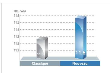
COMPRESSEUR AMÉLIORÉ
